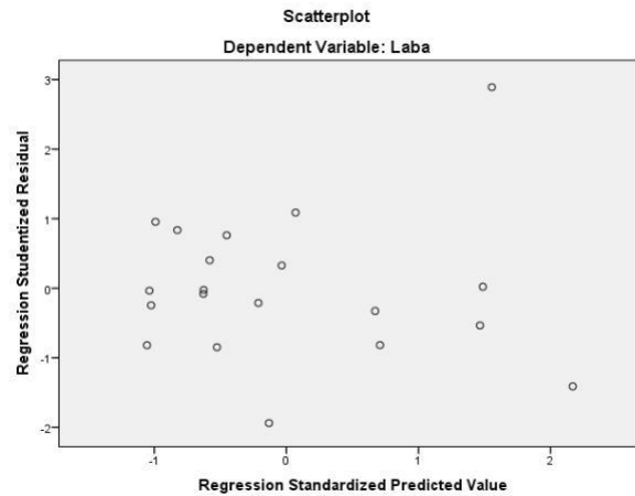
Gambar 6 Heterokedastisitas Scatterplot
