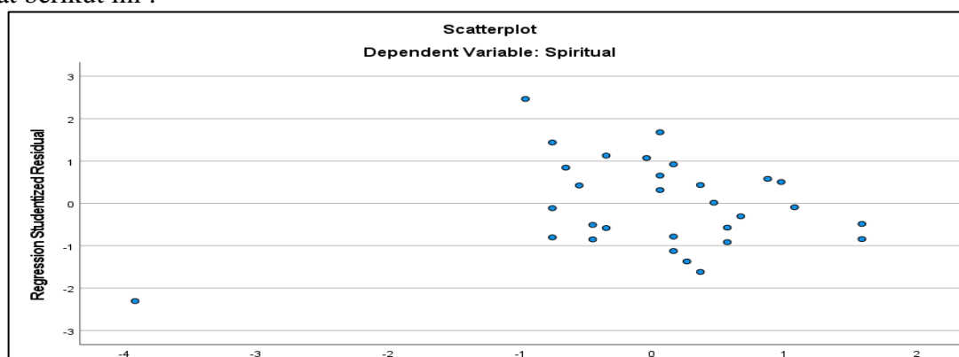
Gambar 1. Uji Heteroskedastisitas
